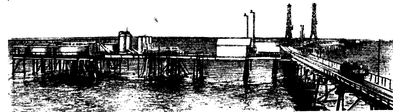
Нефтяные Камни. Одна из секций эстакады.
